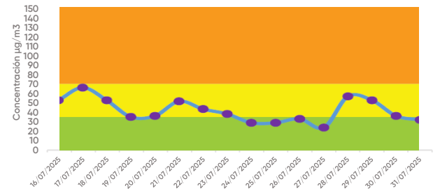
Partículas (PM 2.5 )
