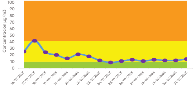
Ozono (O 3 )
