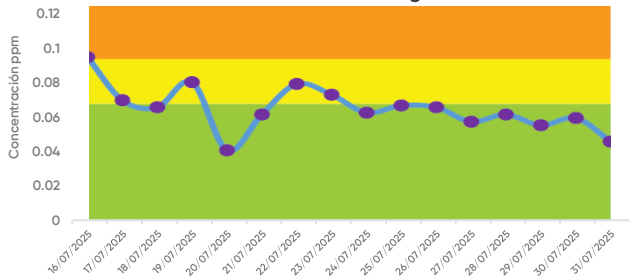
Ozono (O 3 )
